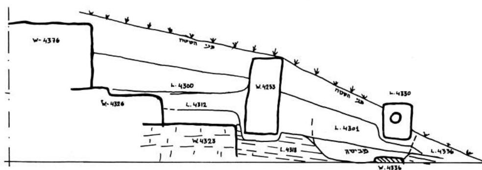
ציור 1: תל דור שטח C; הפביסה והתייחסותה למערכות הביצורים; תכנית וחיתוך
